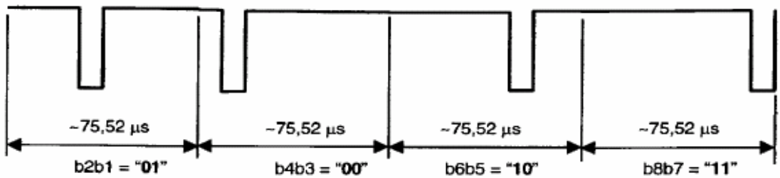
图6 4取1 编码示例
