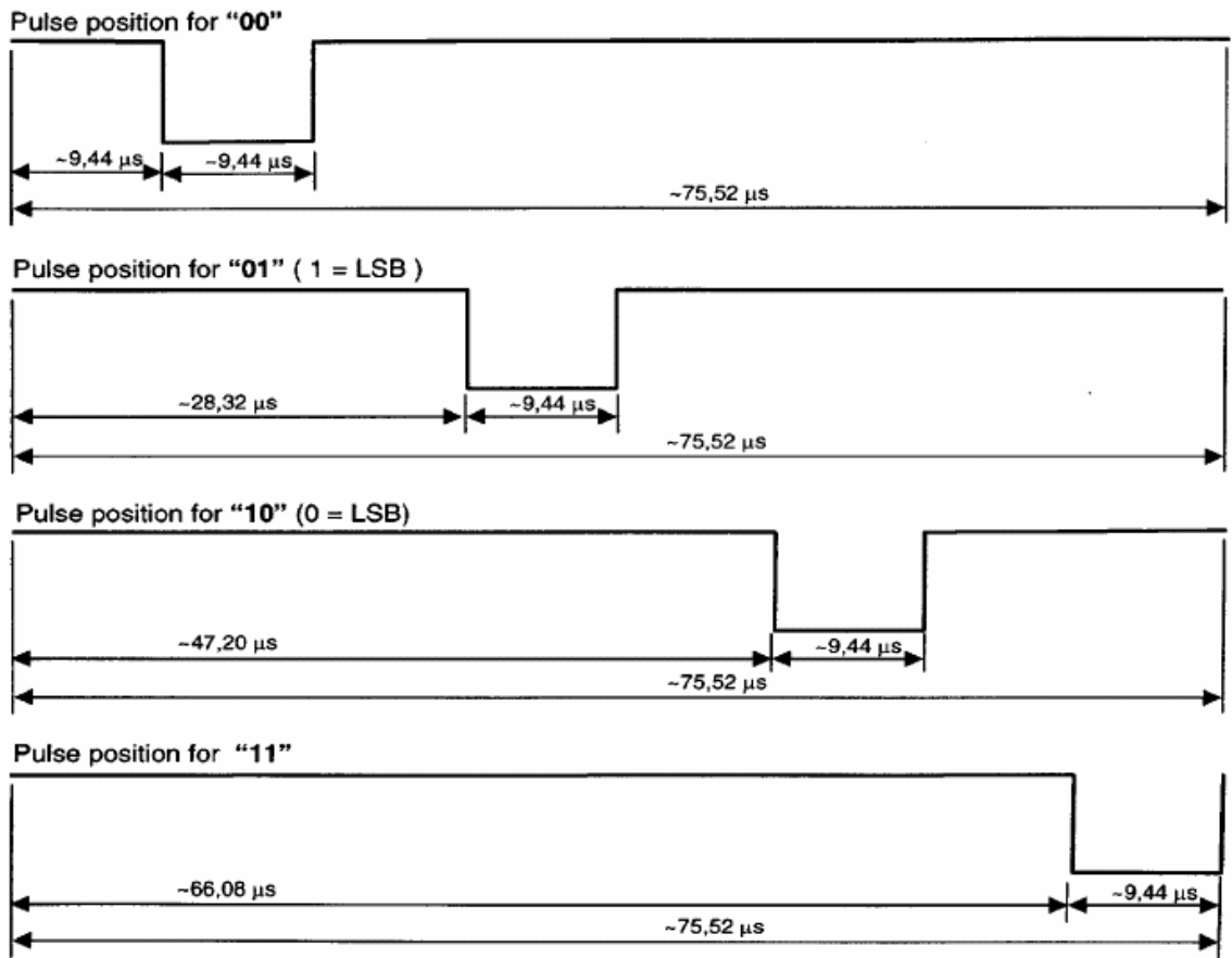
图5 4取1 编码模式
