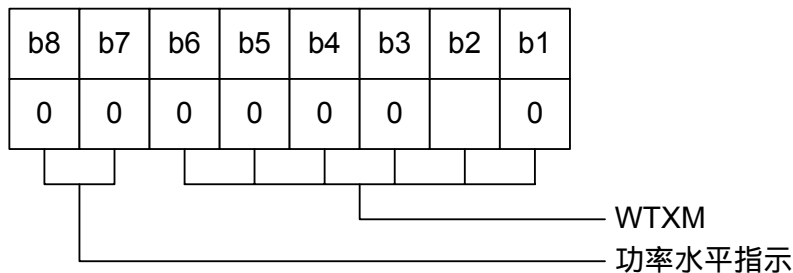
图 3-20 S(WTX)请求的 INF 域编码
