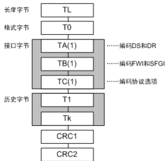
图 3-4 ATS 的结构
