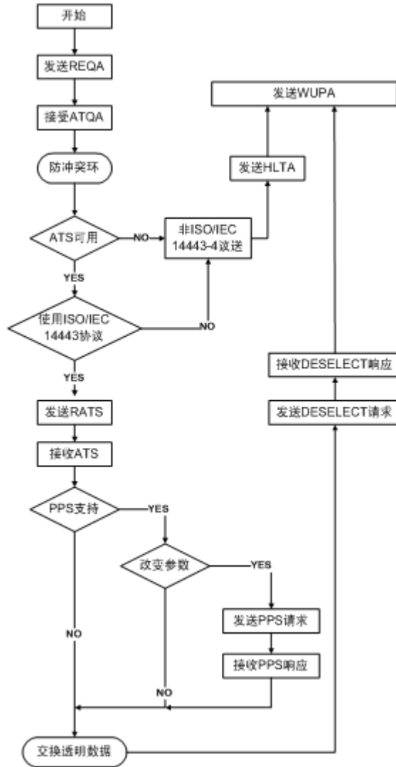
图 3-1 从 PCD 角度看的类型 A PICC 激活
